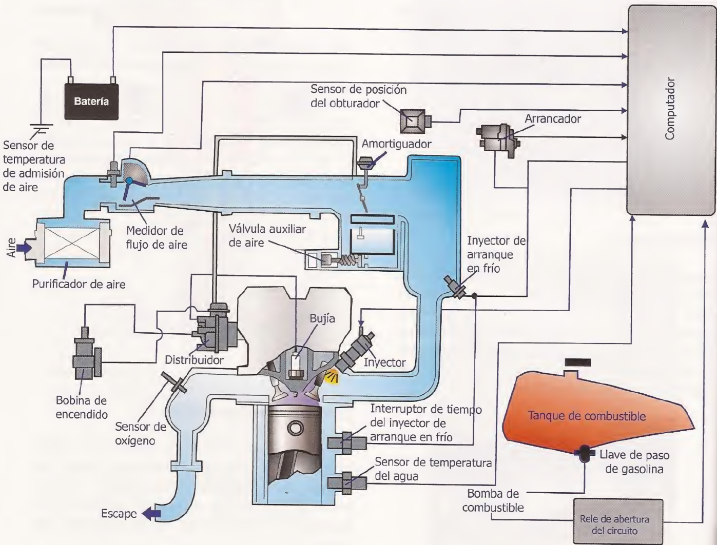
Diagrama del sistema de inyección electrónica
